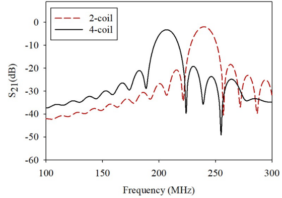
Fig. 9. S_{21} parameter.
